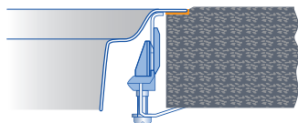
Acciaio inox: installazione filotop
