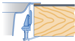
Acciaio inox: installazione sopratop, bordo 1 mm
