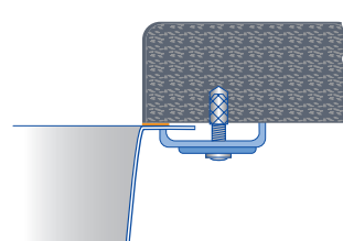
SILGRANIT: vasche sottotop
