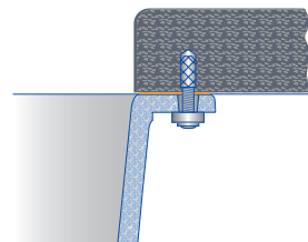
Ceramica: vasche sottotop
