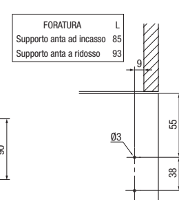
FORATURE ANTA PER SUPPORTO A RIDOSSO
