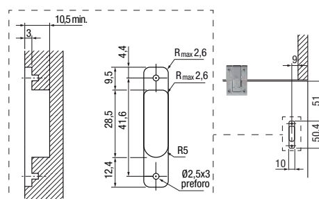
FORATURE FIANCO E SCHIENA PER SUPPORTO AD INCASSO
