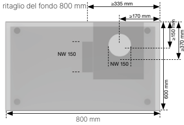
La condotta dell'aria di scarico può essere a destra o sinistra.
