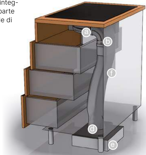
schema d'installazione del sistema di conduzione aria
