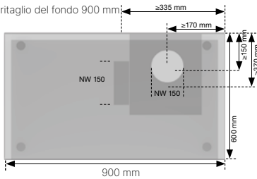
La condotta dell'aria di scarico può essere a destra o sinistra.
